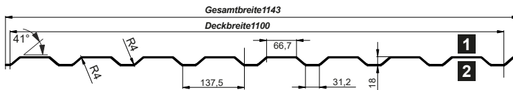
WANDPROFIL
